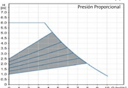
MAGNA3 32-60 (F) (N) MAGNA3 D 32-60 (F)
