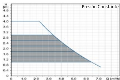
MAGNA3 32-40 (F) (N) MAGNA3 D 32-40 (F)
