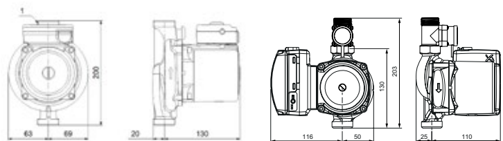
UPA 15-120
