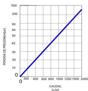
VÁLVULA LIMITADORA
